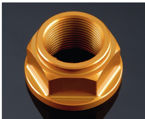
D003 M24X1,5
